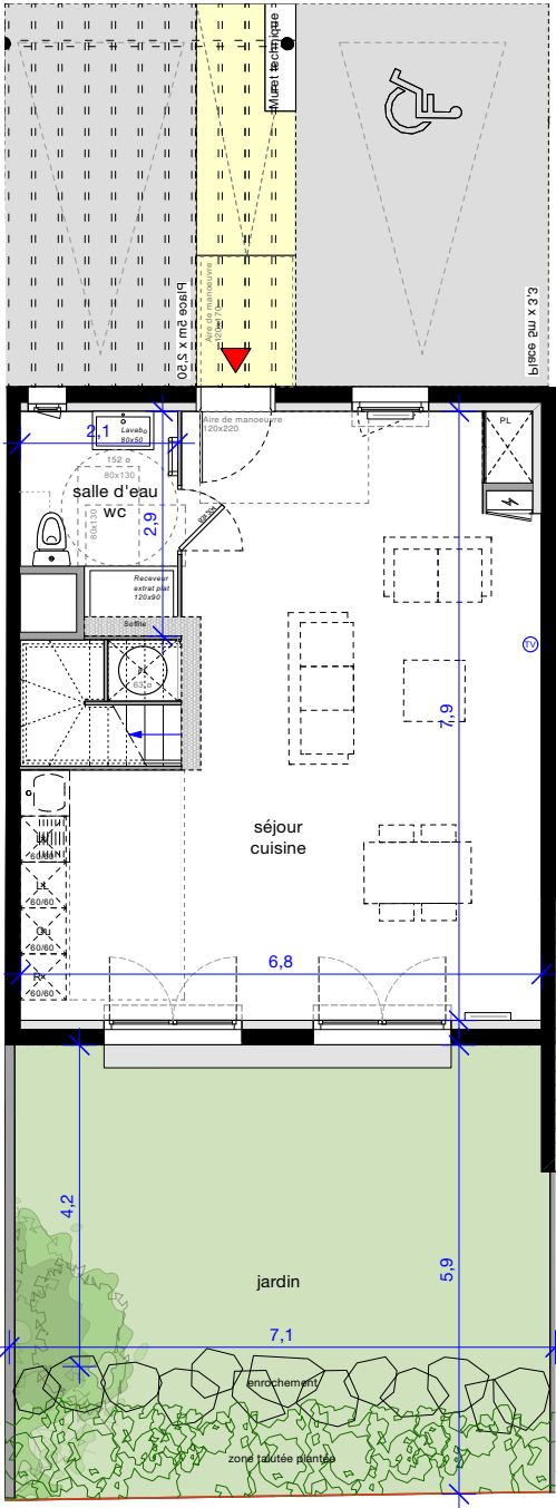
PLAN rez-de-chaussée
