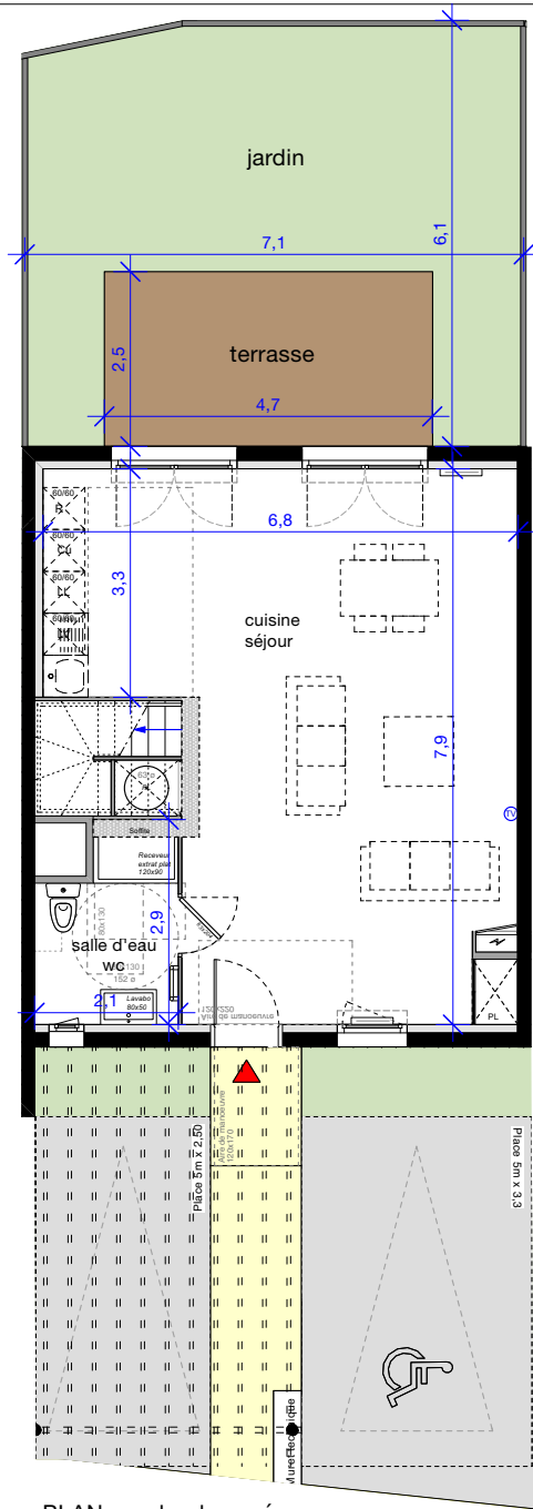
PLAN rez-de-chaussée
